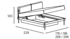
bed frame H 10 with storage box/easy bed Einfassung H 10 mit Bettkasten / Easy bed
