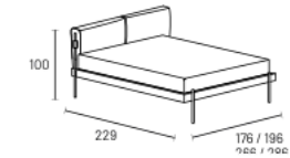
bed frame H 10 with storage box Einfassung H 10 mit Bettkasten
